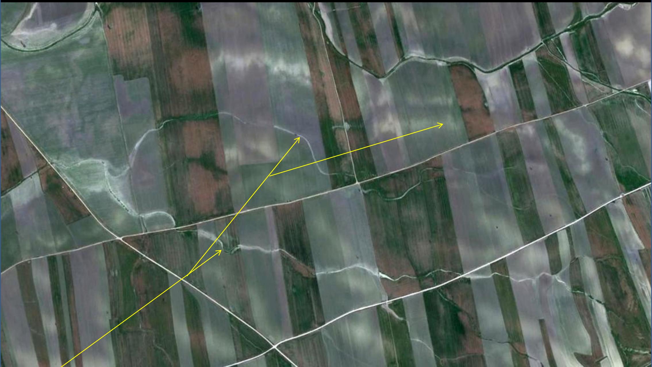
Flujos hídricos bajo los campos agrícolas en las margas del Andaluciense, Mioceno Sup.Terciario. En el NE de Palma del Condado, SW Hoja de San Lucar La Mayor.
