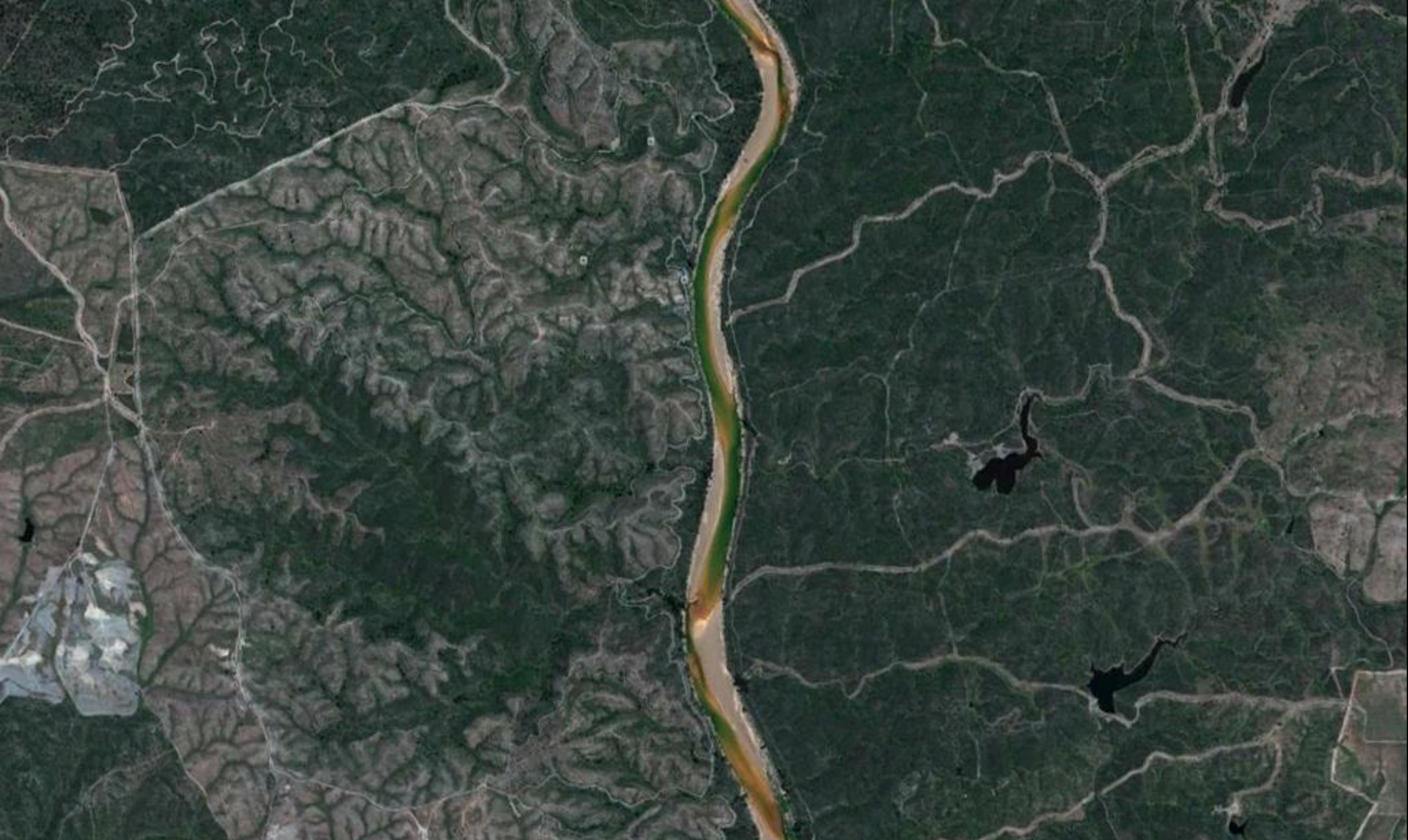
Cambios, por vegetación, en la percepción del drenaje en terrenos del Carbonífero Inf, a ambos lados del Río Odiel. S Barranco Salado y cerrada Embalse de Meca. Hoja de Gibraleón.
