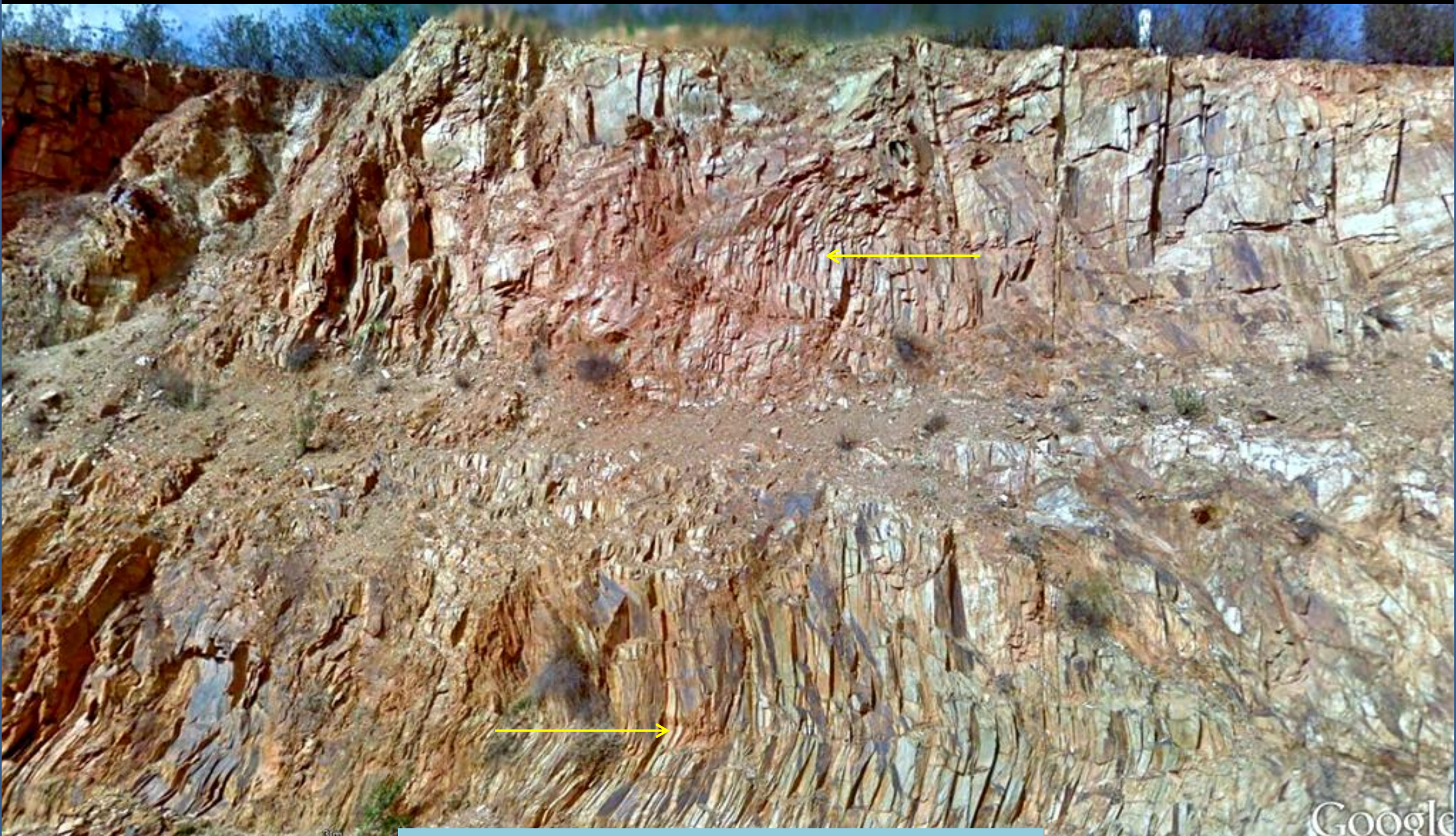
Pizarras basales del Viseiense Sup. Dinantiense, Carbonífero Inf. Entre el Río Tinto y Arroyo Corumbel. NE Hoja de La Palma del Condado. Zona de cizalla?
